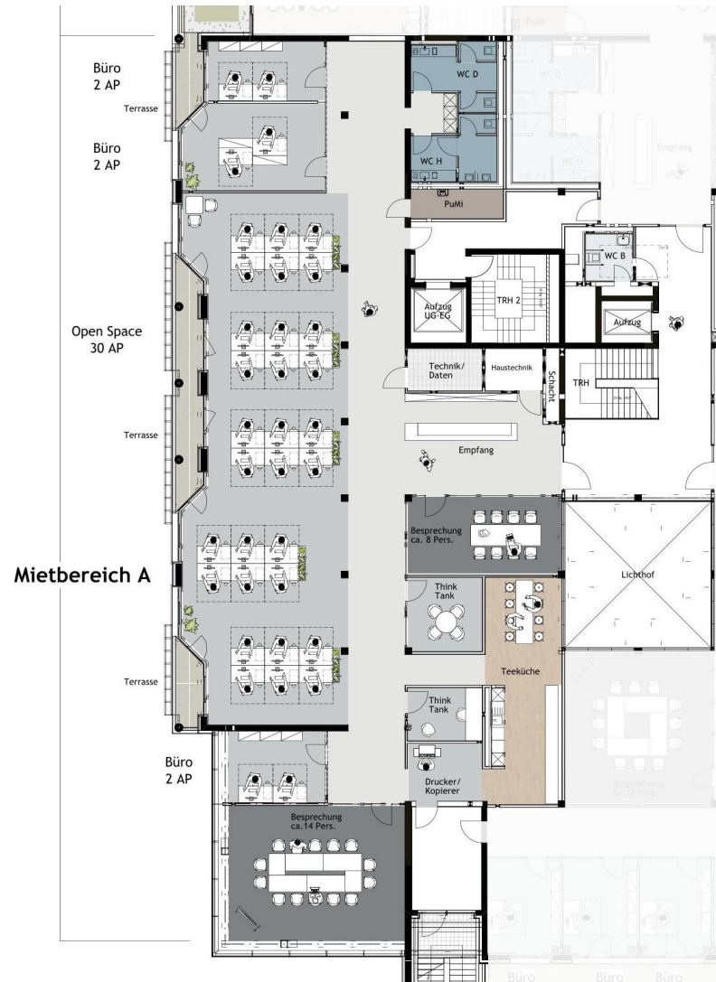
Beispielhafte Belegungsplanung mit ca. 37 Arbeitsplätzen
