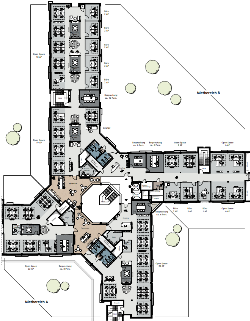
2.OG Regelgeschoss mit Mietbereich A (ca. 51 Arbeitsplätze) und Mietbereich B (ca. 74 Arbeitsplätze) sternhöhe | Haus 2 | Epplestraße 225 | 70567 Stuttgart
