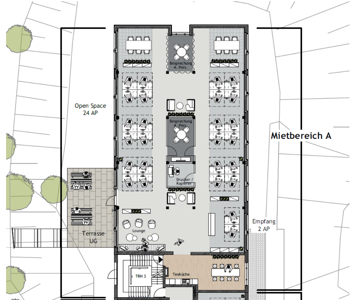
Gartengeschoss mit ca. 26 Arbeitsplätzen
